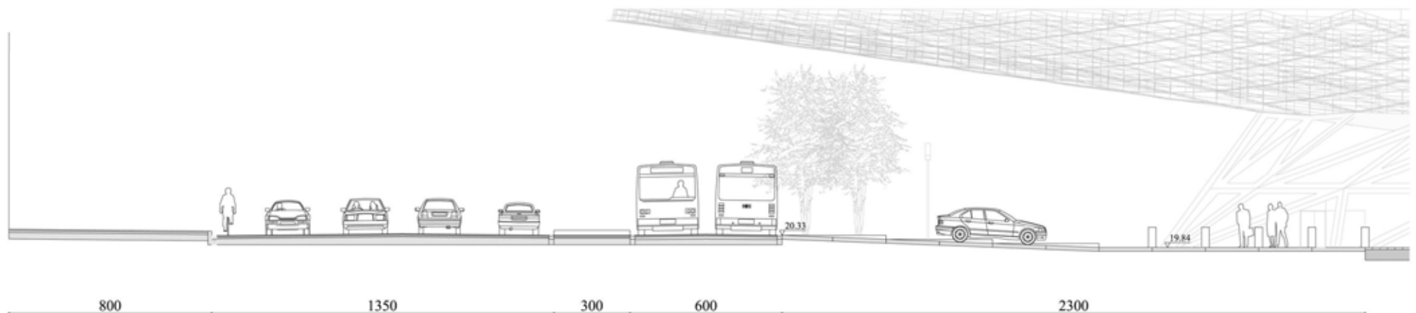
COUPE/SNEDE EE
